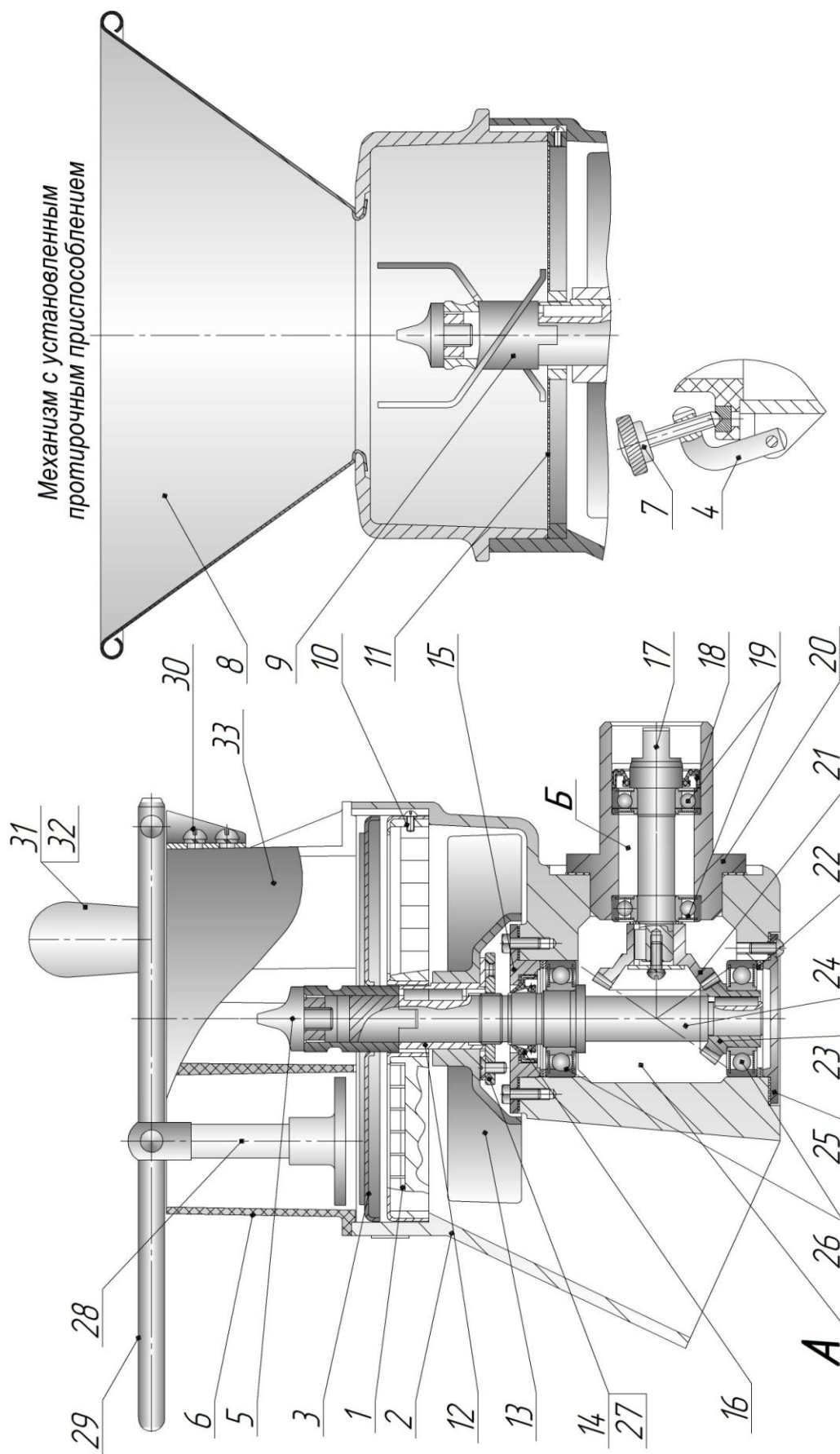
Рисунок – 4 Механизм ошцезательно – протирачный
